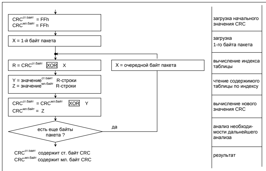
Рисунок 3-8. Рекомендуемый алгоритм расчета контрольной суммы.
