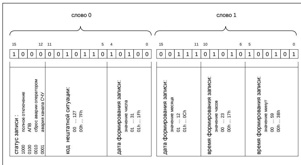
Рисунок 4-8. Структура записи архива аварий.
