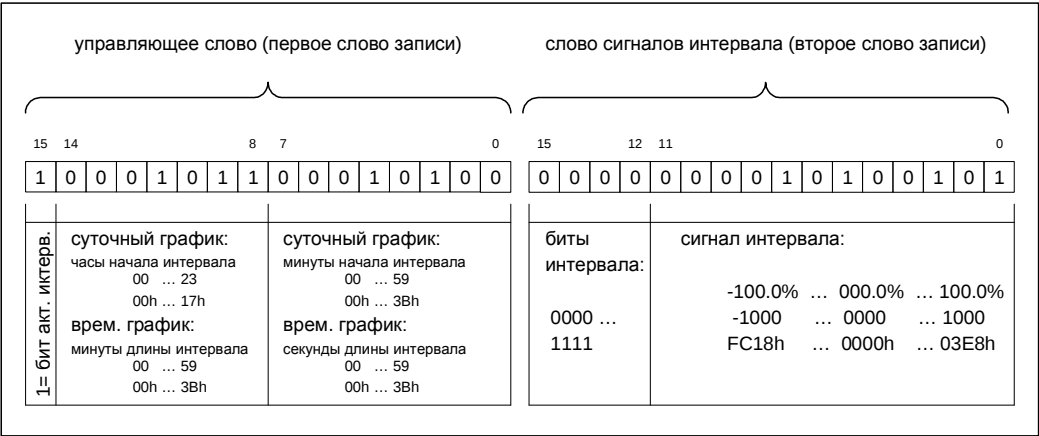
Рисунок 4-12. Структура записи временного/суточного графика.
