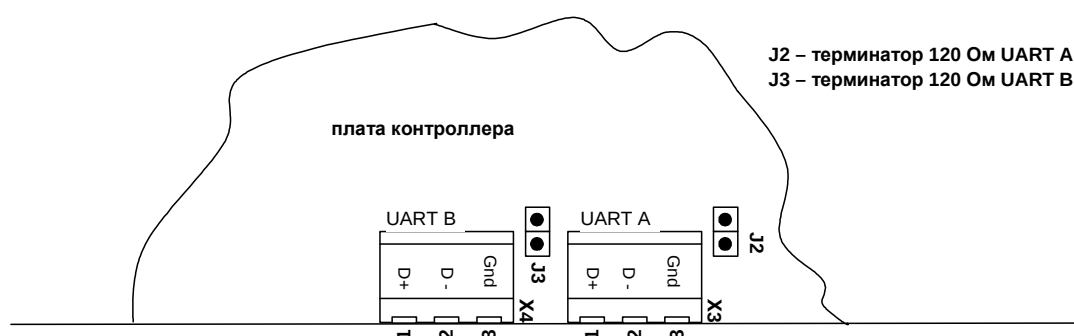
Рисунок 2-1. Расположение разъемов подключения RS485.
