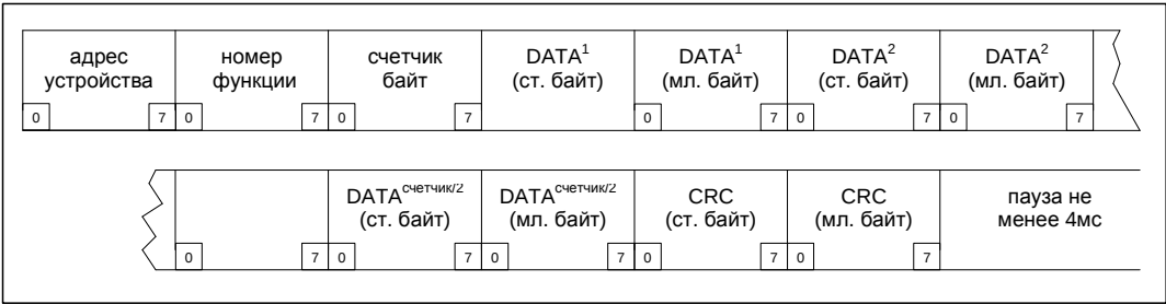
Рисунок 3-4. Штатный ответ на запрос чтения.
