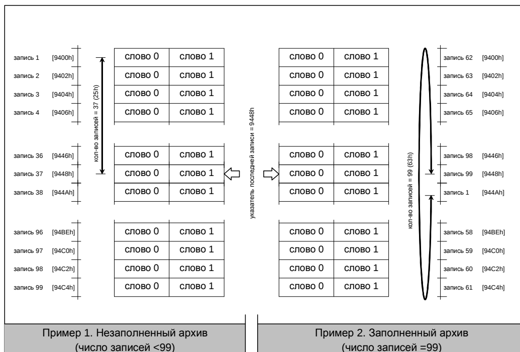
Рисунок 4-9. Структура архива аварий.
