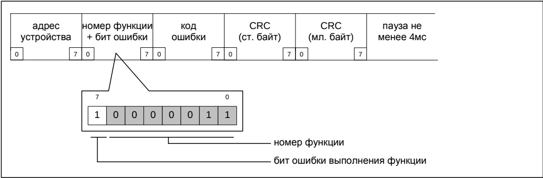
Рисунок 3-5. Ответ на неправильный запрос чтения/записи.
