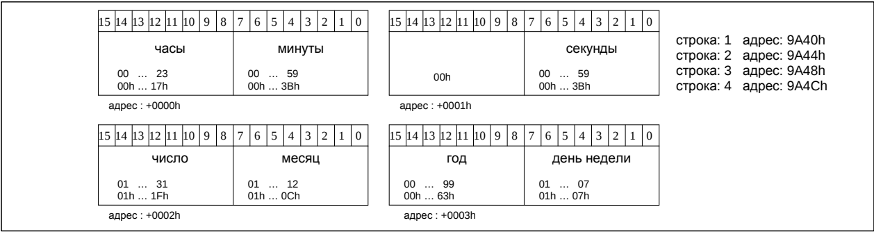
Рисунок 4-5. Структура записи буфера «дата/время».
