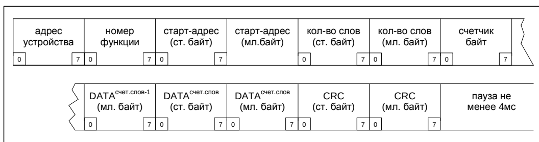
Рисунок 3-6. Последовательность запроса записи.
