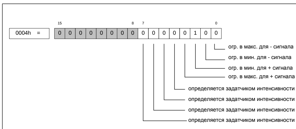
Рисунок 4-2. Представление шестнадцатеричного параметра.
